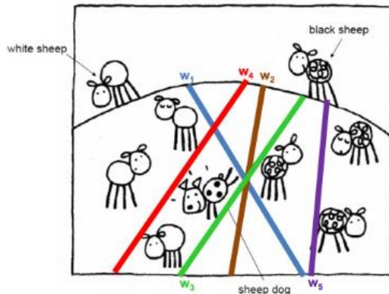
Linear SVM
