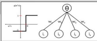
F. Rosenblatt
