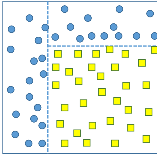
Case 2
